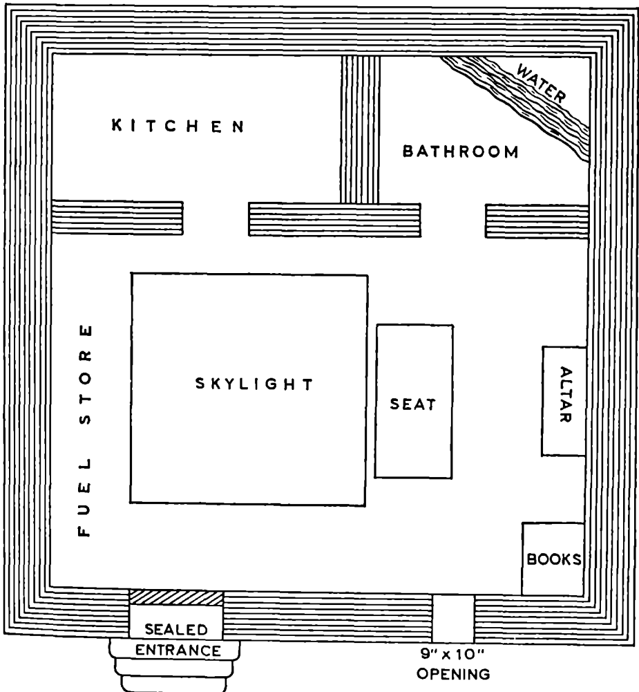
Lung-gom Hermitage (ground-plan)
